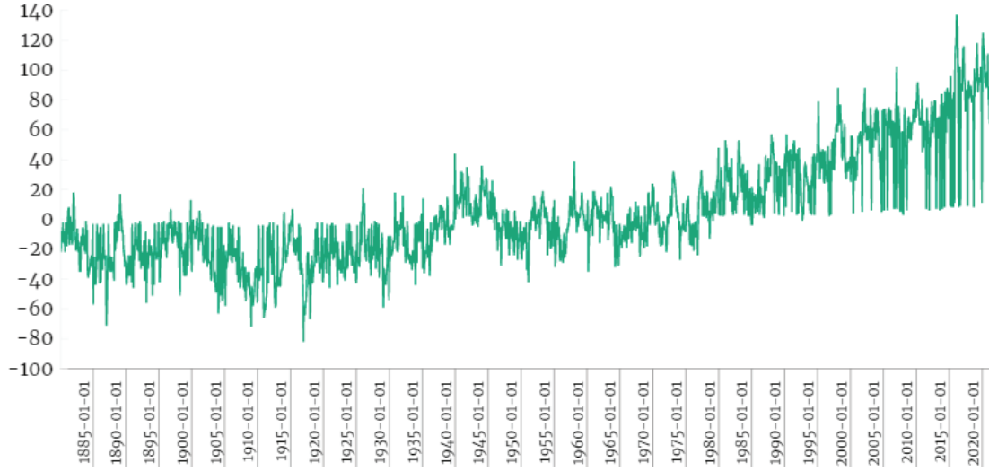
Grafik 8. Küresel Isınma: Aylık Sıcaklık Anomalisi (1880-2021)
