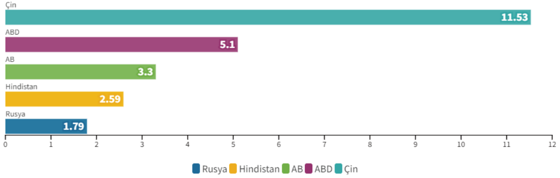
Grafik 9. Grafik: Gelişmiş Ülkelerdeki Toplam Karbon Emisyonu (Megaton)
